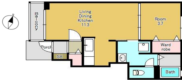
1階 タイプ 37.13㎡
